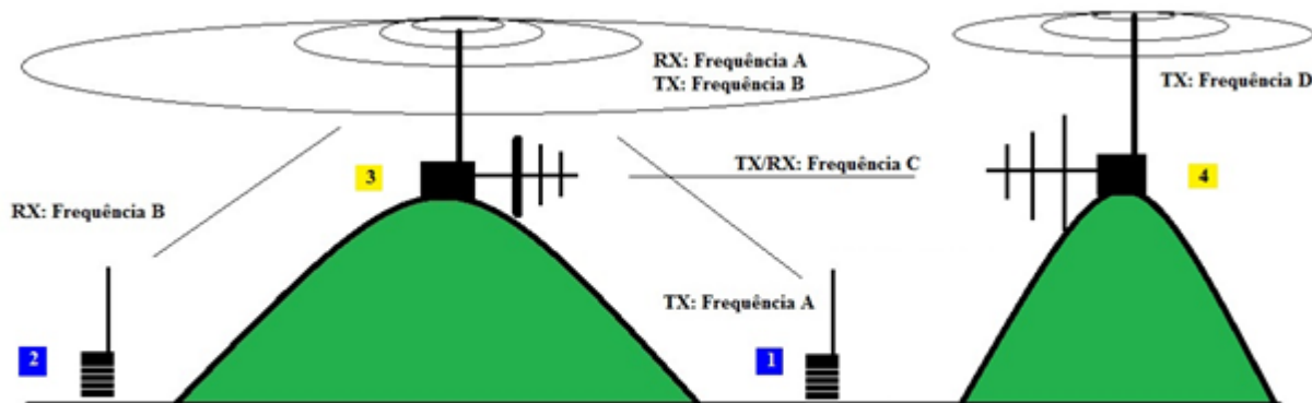
Esquema do funcionamento de uma Repetidora
